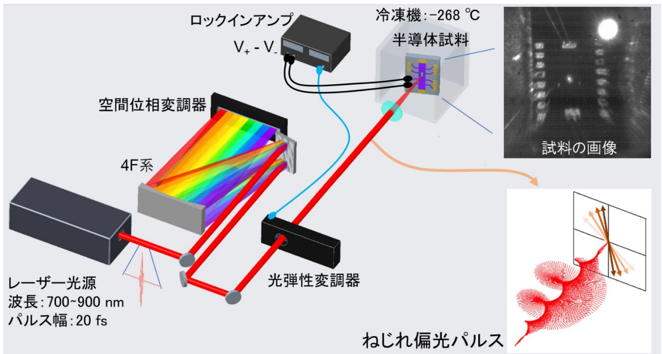
図 2 本研究で開発された光電場波形の制御機構。レーザー光は周波数及び進行方向に直行した 2 成分ごとに空間位相変調器の各ピクセルへ導かれ、それぞれ個別に位相を制御することで任意の波形を整形できます。この技術でレーザー光の電場の振動方向が回転していくねじれ偏光パルスを生成しました。
